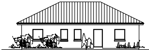
ANSICHT EINGANGSSEITE
